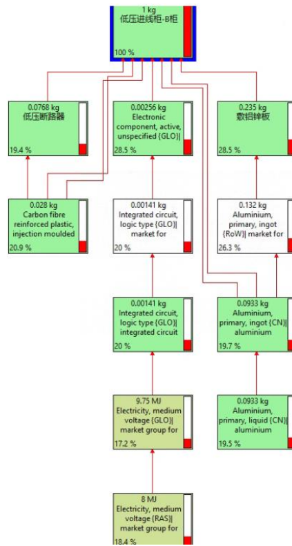
生命周期碳足迹结果网状结构图低压成套开关设备（Blokset）
